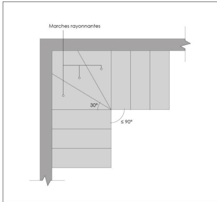
Illustration 4 Marches rayonnantes
