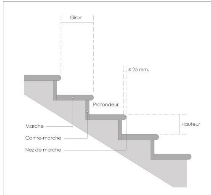
Illustration 1 Hauteur de marche, giron et profondeur de marche
