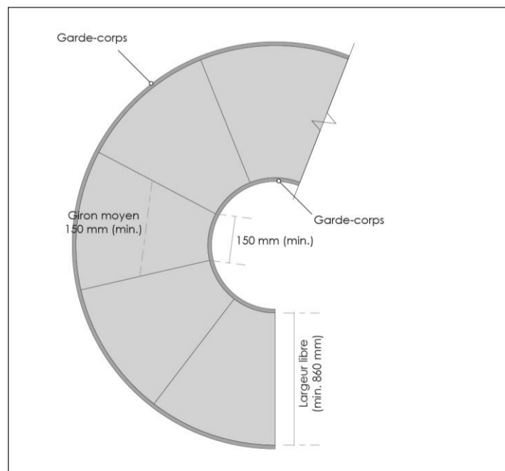
Illustration 3 Escalier hélicoïdal
